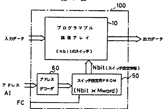
本発明の一実施例のブロック図 第2図
